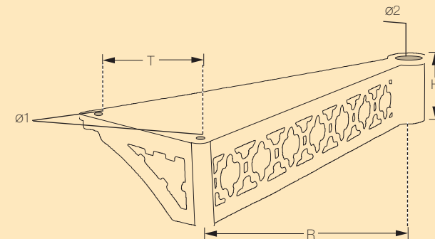
Zierrücker mit Gewindestange M12
